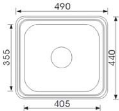
YH121C (490×440×180mm)
